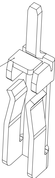
封口端子图
